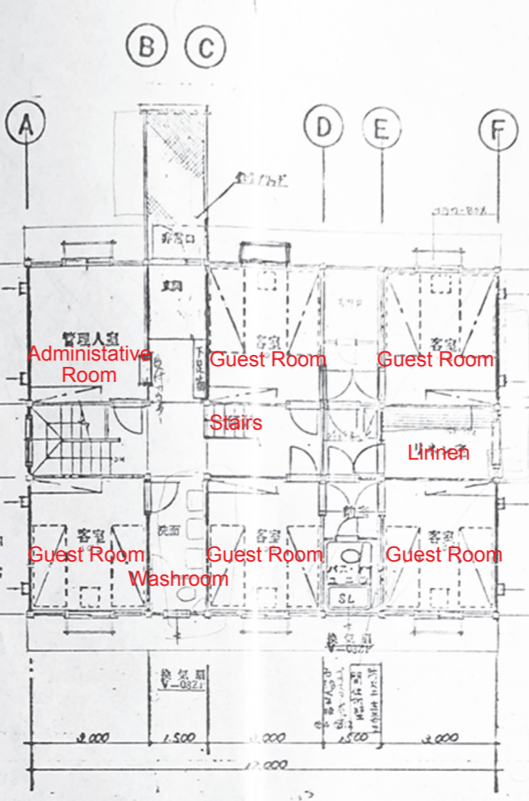
1F 平面図 1F
