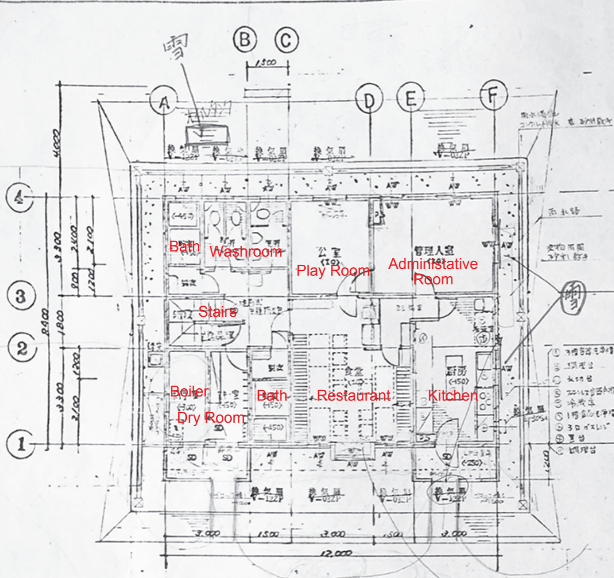
地下室平面図 BF
