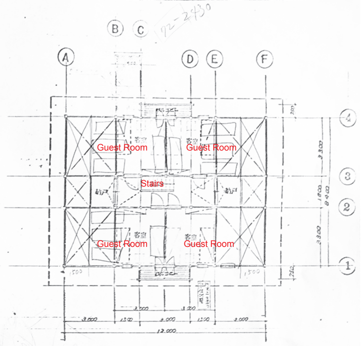
2F 平面図 2F
