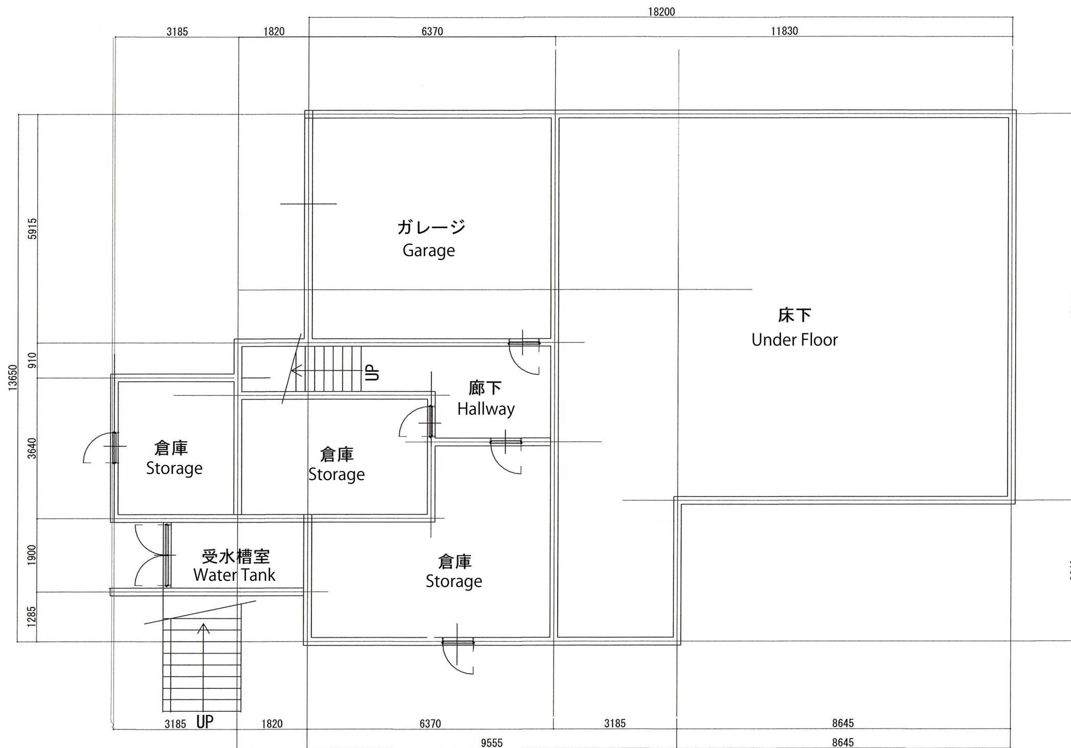
地階平面図 S=1/100
