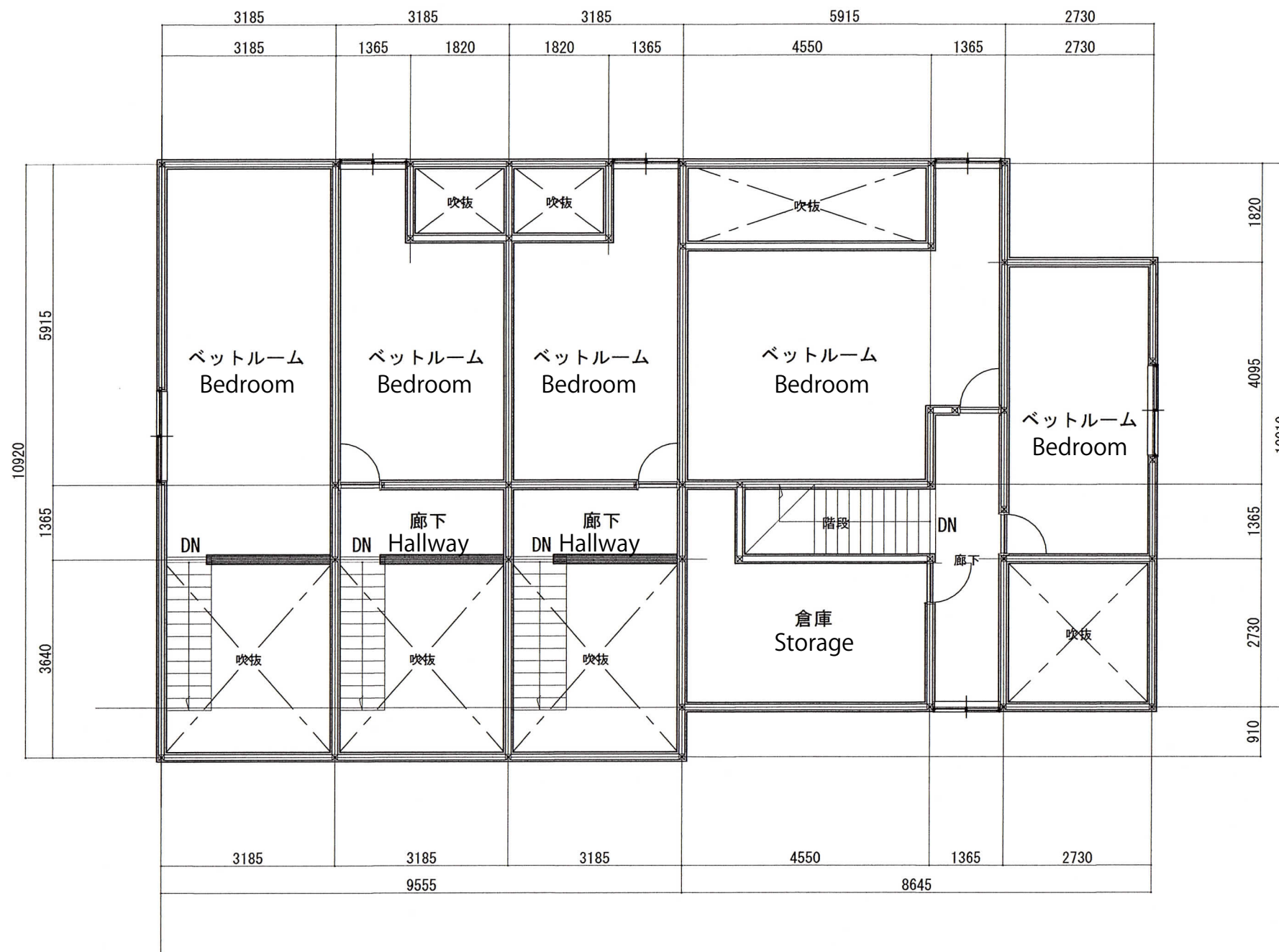
小屋裏 S= 1/100
