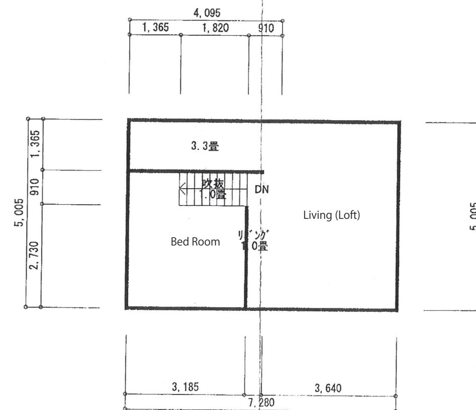
2階 縮尺 1/100
