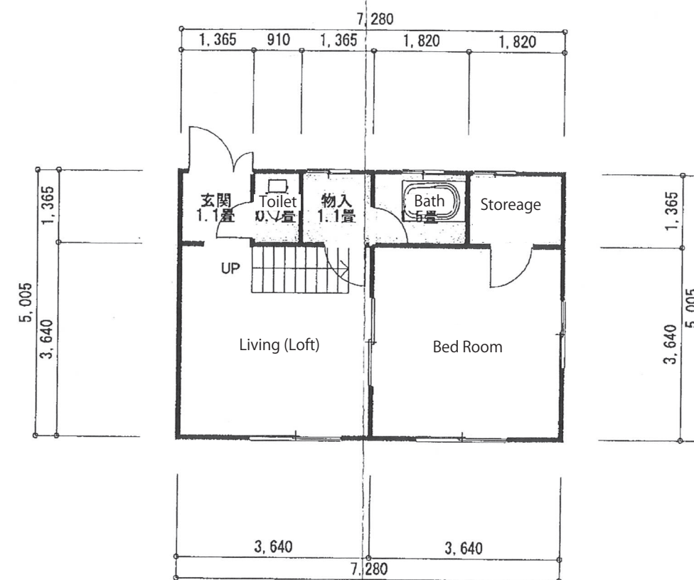
2階 縮尺 1/100
