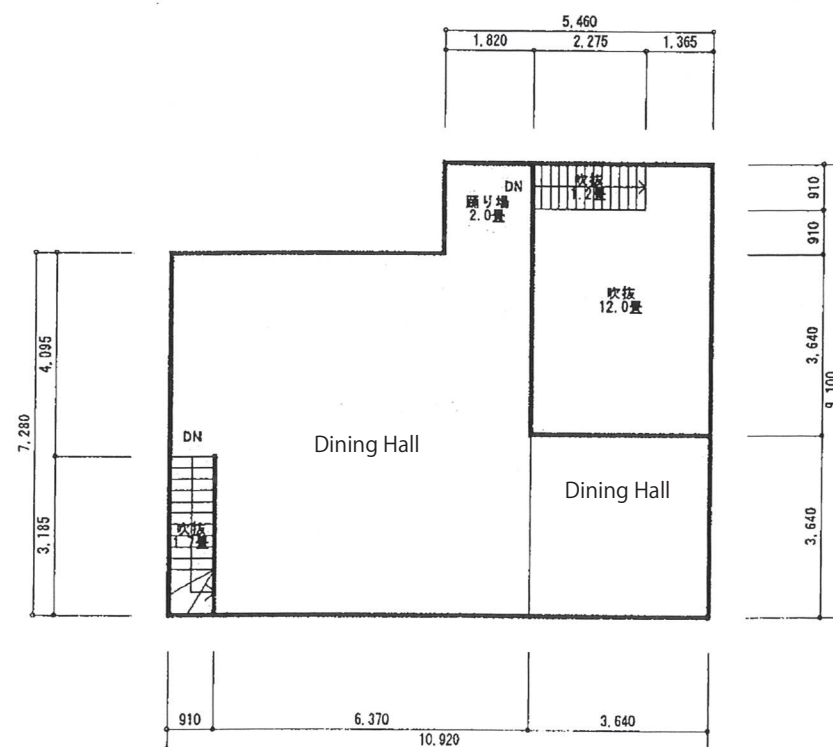
2階 縮尺 1/150
